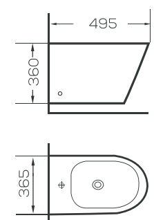
ESQUEMA (mm)
